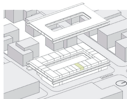
2. Obergeschoss
